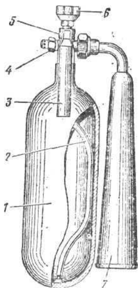
Рис. 43. Устройство углекислотного огнетушителя; 1 — баллон; 2 — сифонная трубка; 3 — рукоятка; 4 — предохранитель; 5 — вентиль; 6 — маховичок; 7 — раструб
